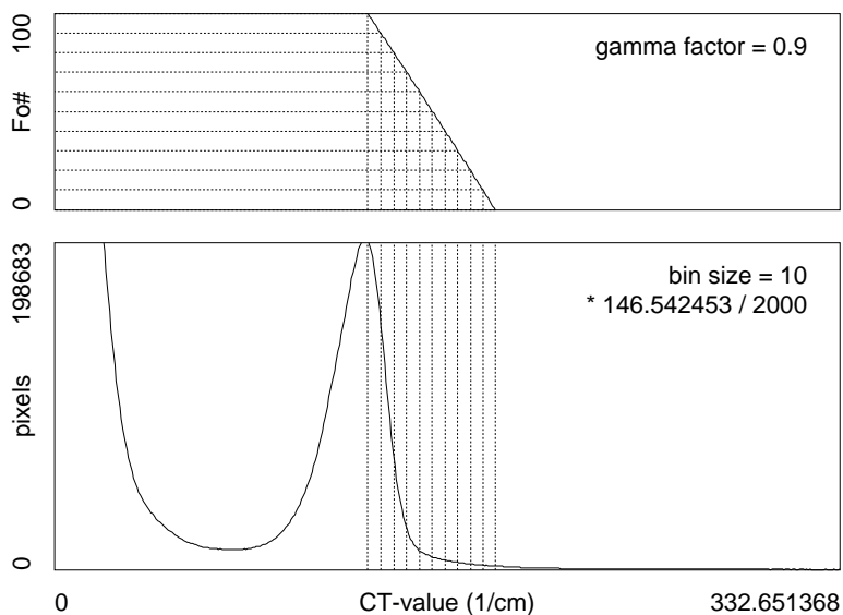
041002b : 7.098 keV
