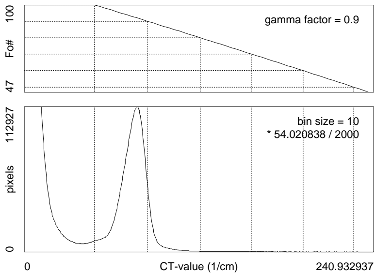
041002c : 10 keV
