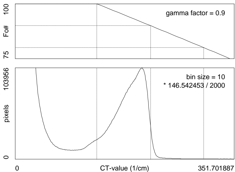
041002a : 7.124 keV
