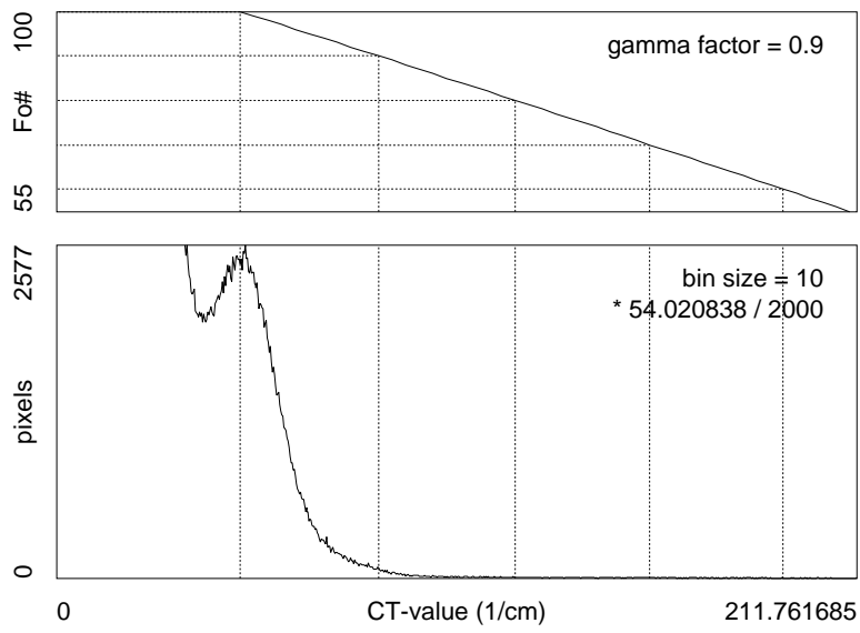
041002g : 10 keV
