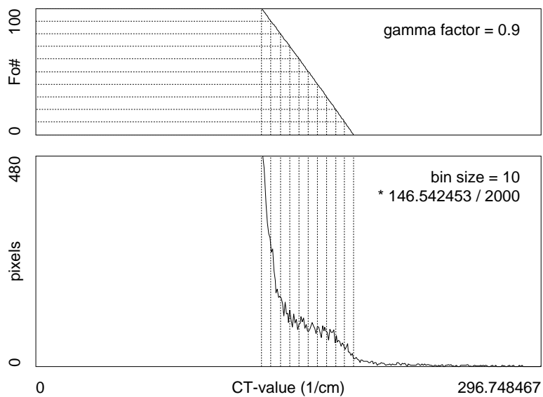
041002i : 7.098 keV
