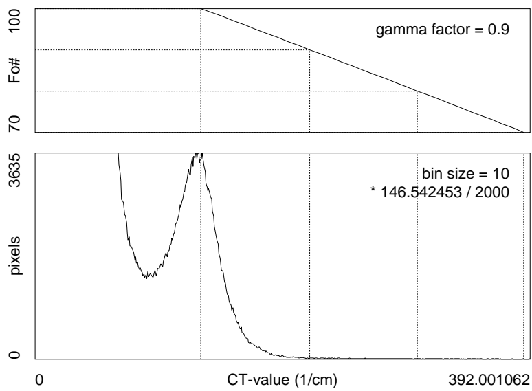
041002h : 7.124 keV
