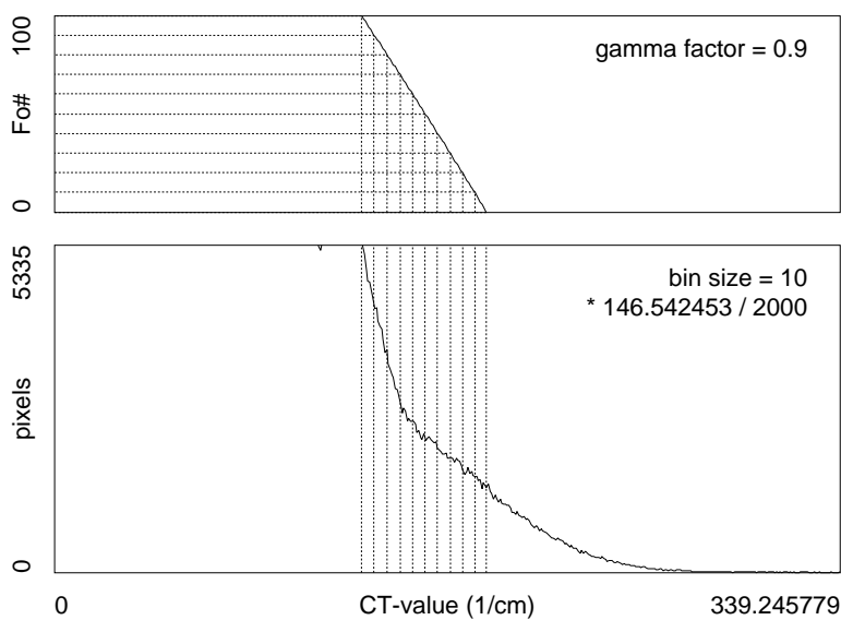
041002k : 7.098 keV
