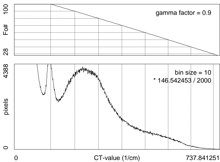
041002j : 7.124 keV
