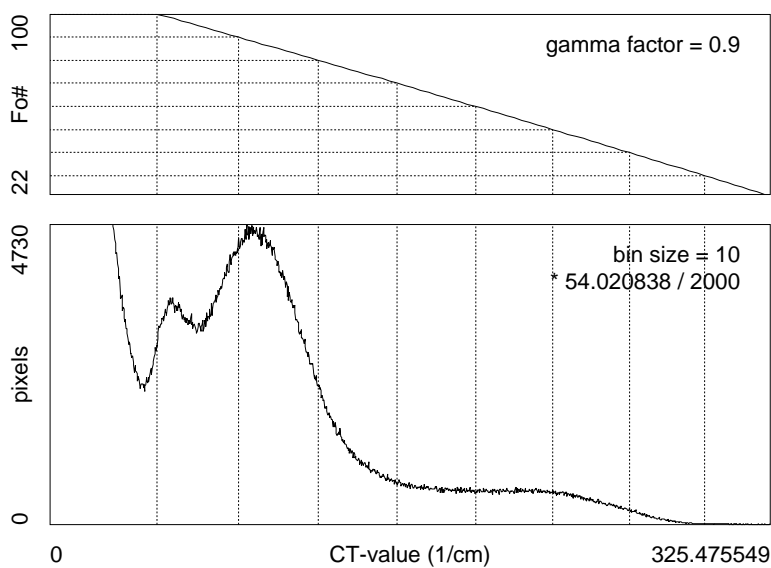
041002l : 10 keV
