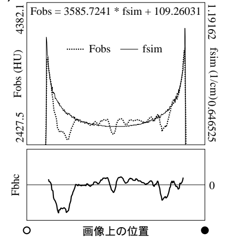
(d) 線分上の CT 値プロファイル
