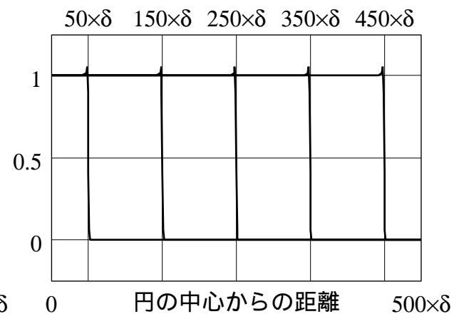
Chesler フィルタ
