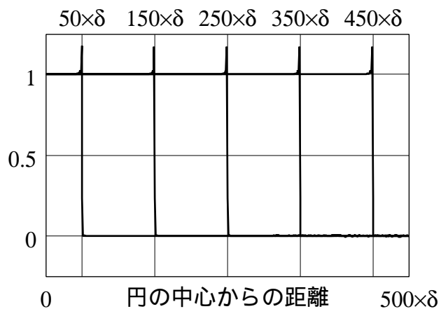
Ramachandran フィルタ
