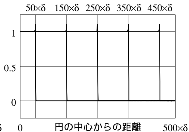
Shepp フィルタ
